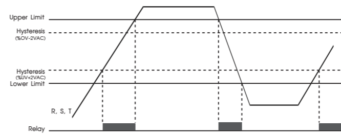
การทำงานแบบ 3-Phase Under and Over Voltage Protection
