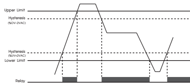
การทำงานแบบ 1-Phase Under and Over Voltage Protection
